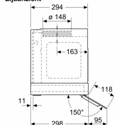
Afmeting in mm Zijaanzicht
