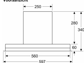
Afmeting in mm Vooraanzicht
